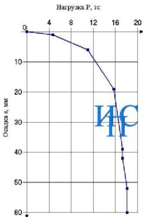
Рис. 2. Графики зависимости осадки
