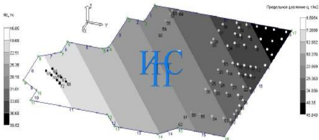
Рис. 1. Пример расчета давления на грунт в подошве фундамента, усиленного сваями Titan
