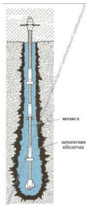
Рис. 3. Разрез сваи Titan
